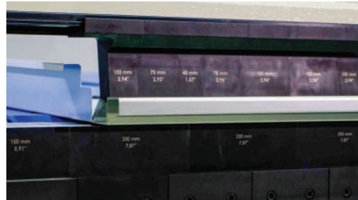
UP BEND / YUKARI YÖNLÜ BÜKÜM
